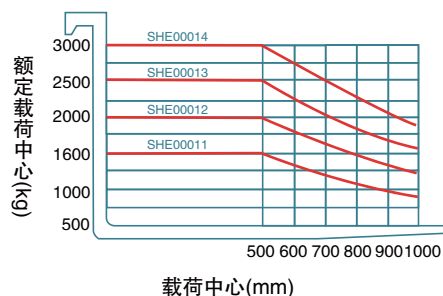
四支点平衡重式蓄电池叉车负荷曲线图
